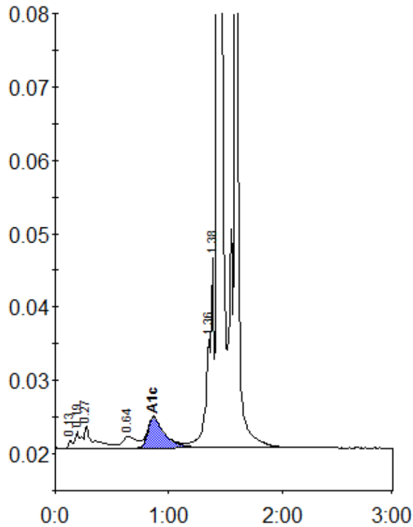
Peak table - ID: 10666724
